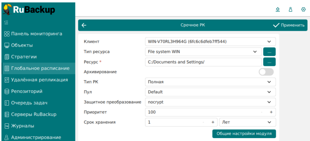
Рисунок 17. Окно настройки Срочного резервного копирования
