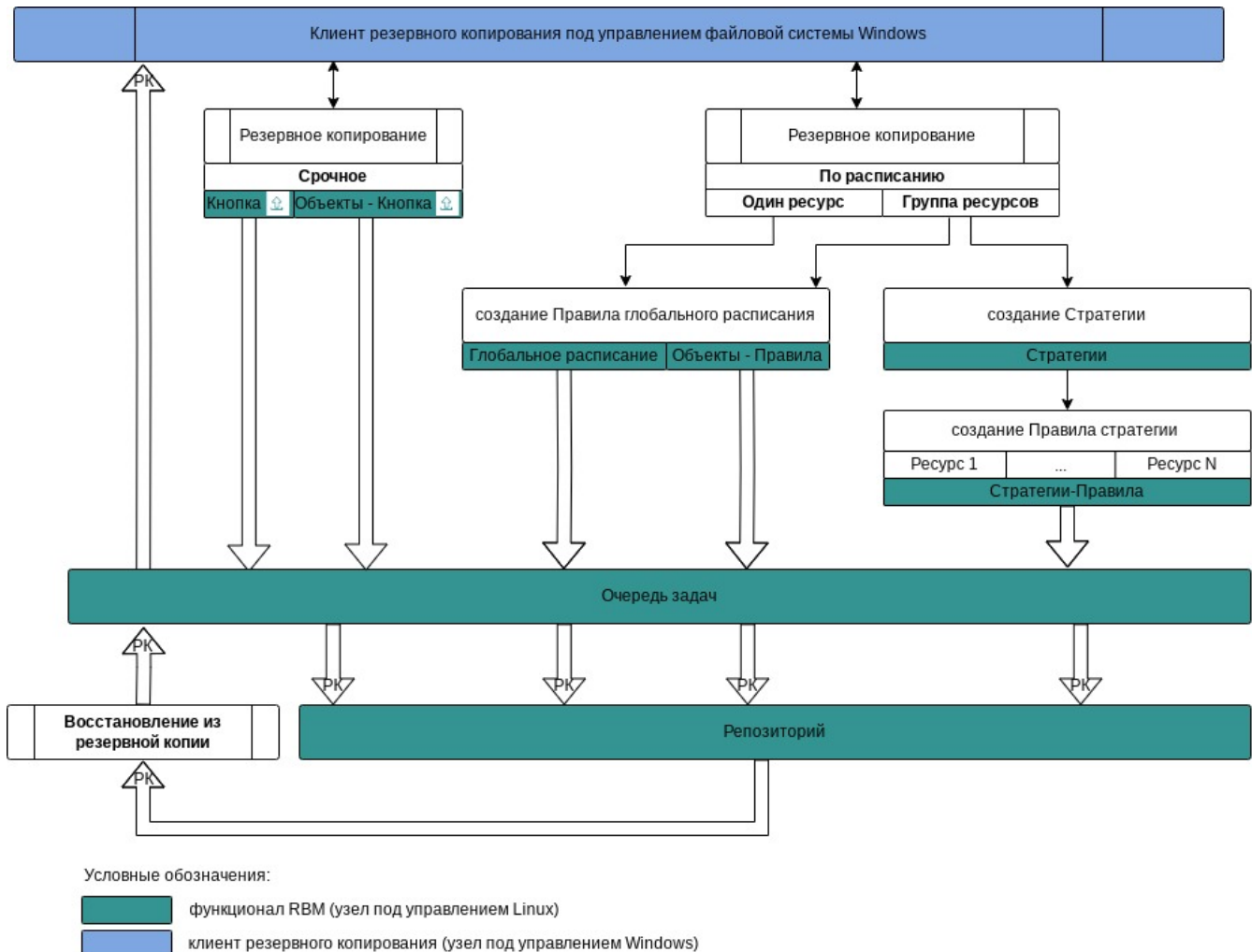
Рисунок 1. Структурная схема резервного копирования и восстановления файловой системы Windows
