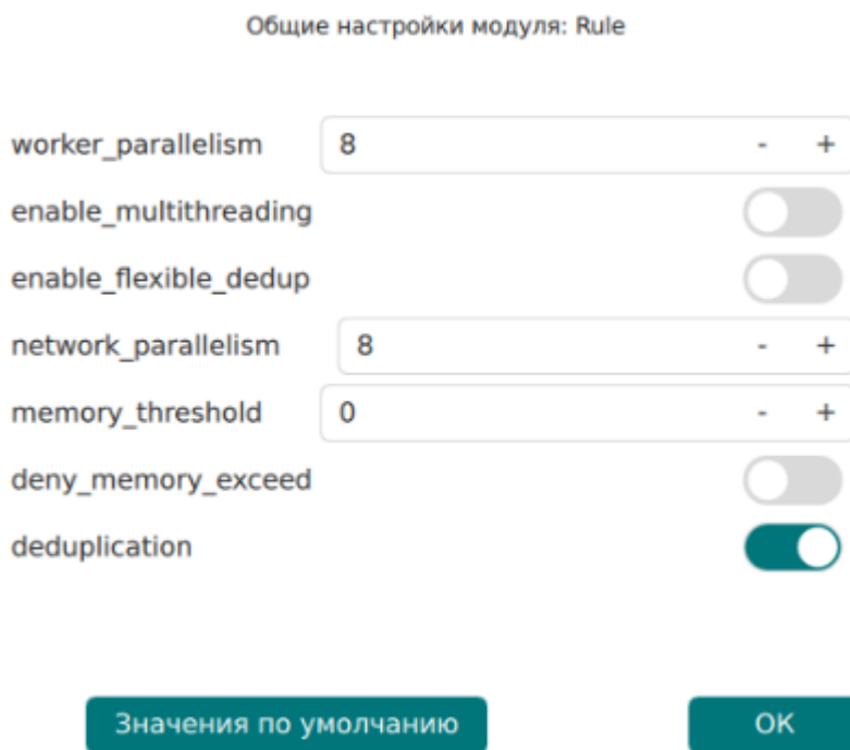
Рисунок 26. Окно Общие настройки модуля (значения по умолчанию)
