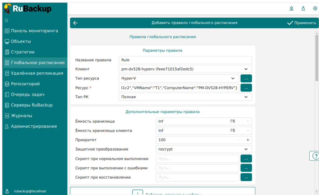
Рисунок 7. Добавление правила глобального расписания
