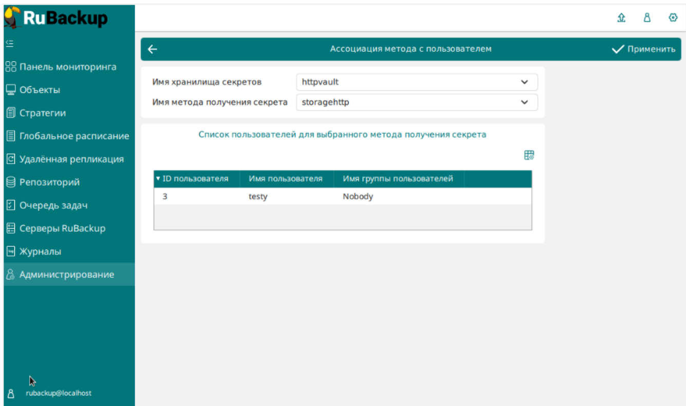
Рисунок 16. Сохранение результата
