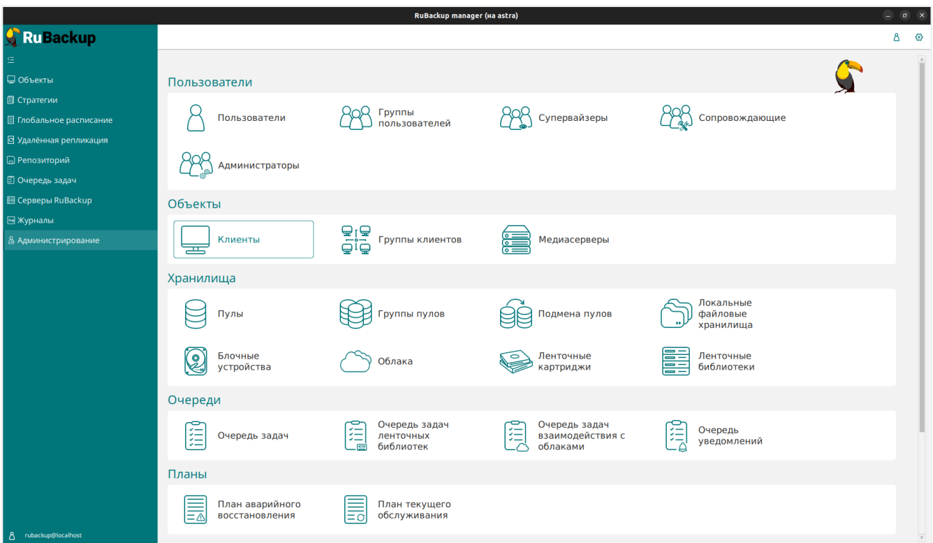
Рисунок 8. Раздел "Администрирование"
