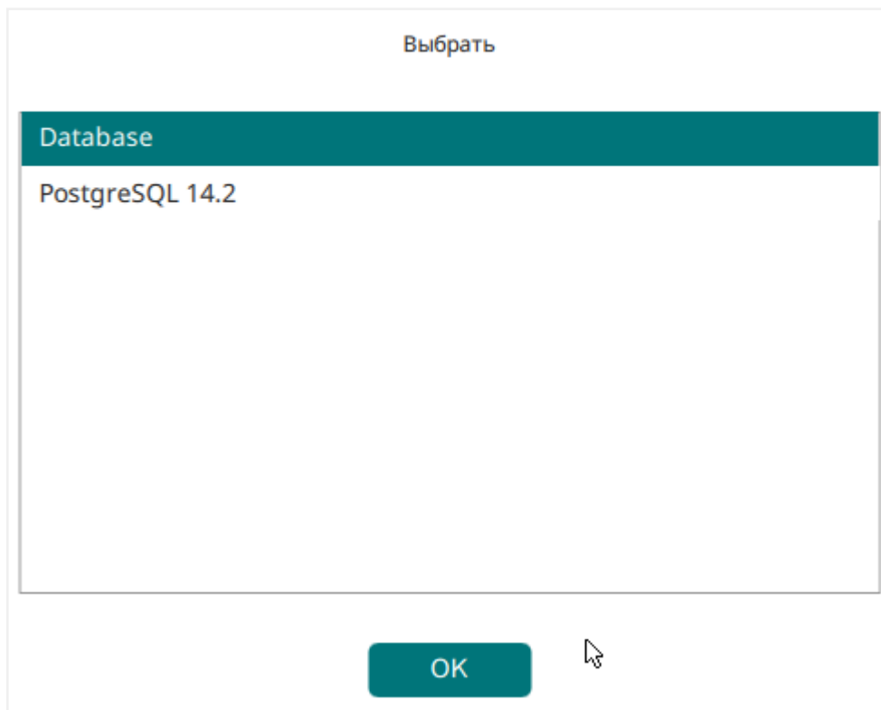
Рисунок 47. Проверка конфигурации
