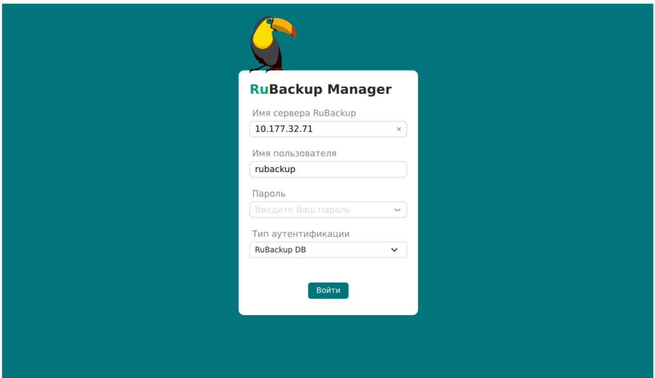
Рисунок 7. Запуск RBM
