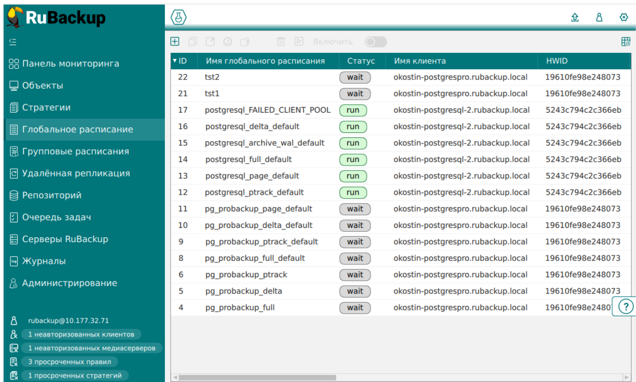
Рисунок 17. Глобальное расписание
