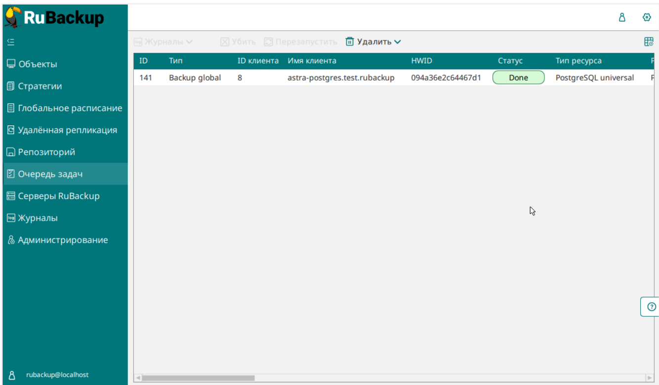
Рисунок 27. Очередь задач
