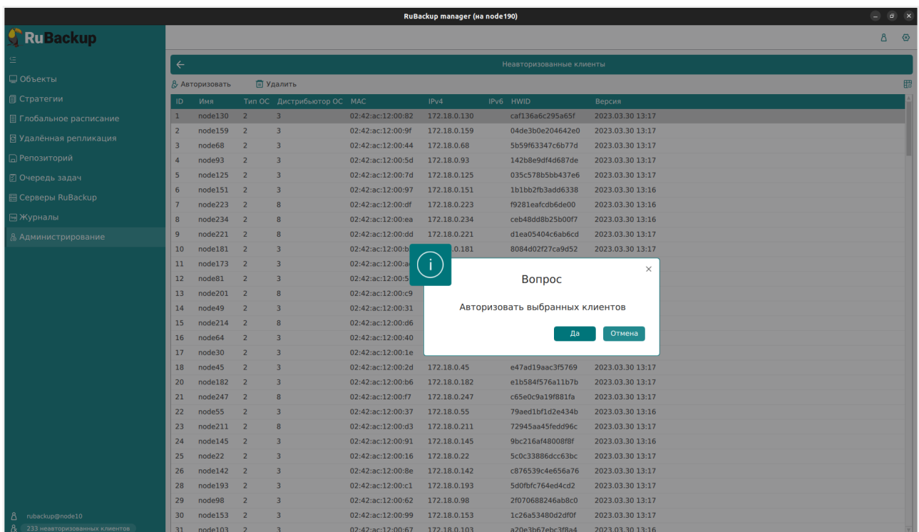
Рисунок 11. Авторизация клиентов
