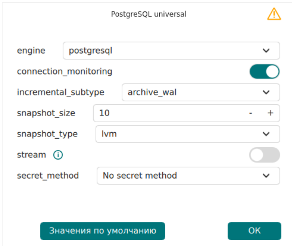
Рисунок 19. Предупреждение
