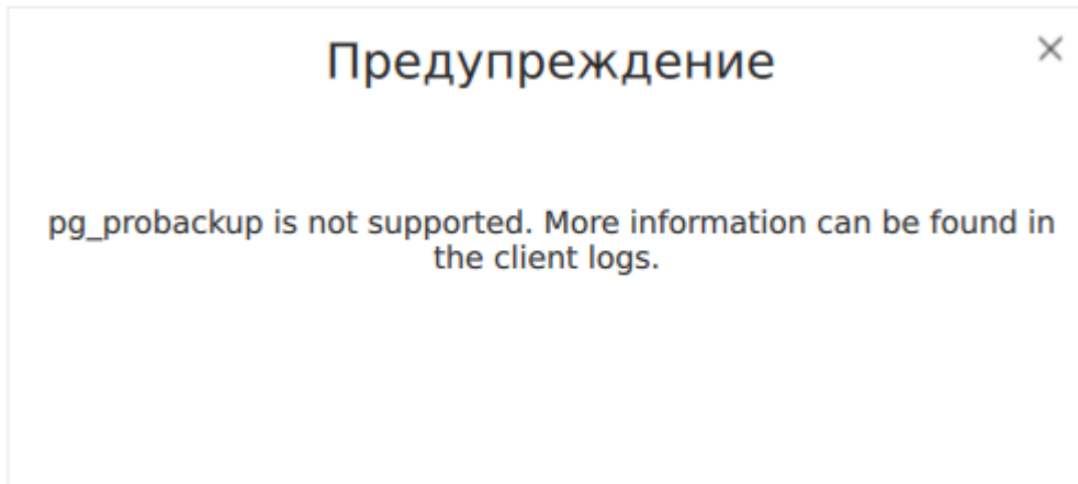
Рисунок 20. Подробная информация
