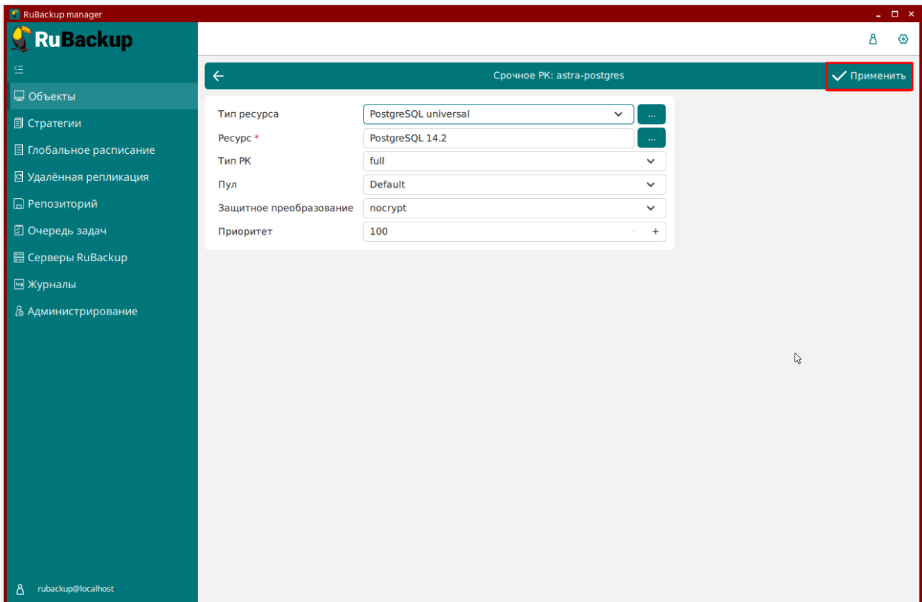
Рисунок 26. Кнопка "Применить"
