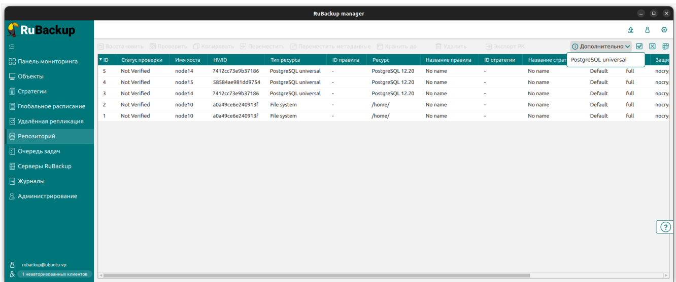
Рисунок 30. Раздел «Репозиторий»
