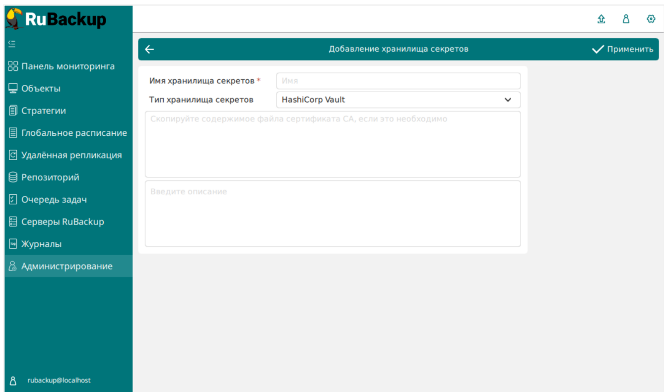
Рисунок 14. Сохранение настроек
