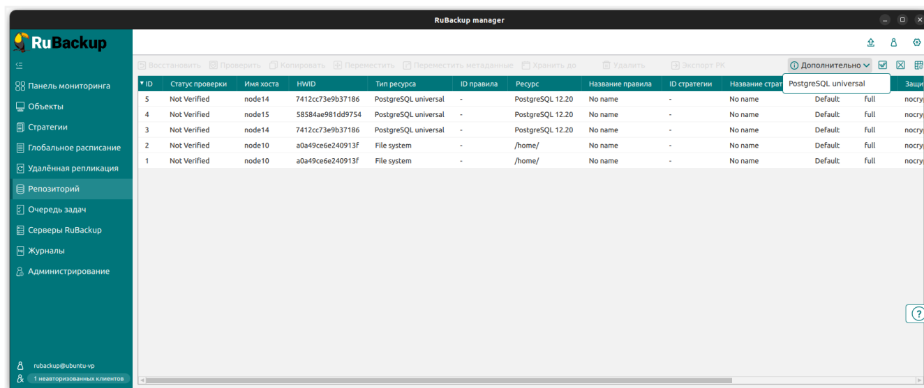
Рисунок 27. Раздел «Репозиторий»
