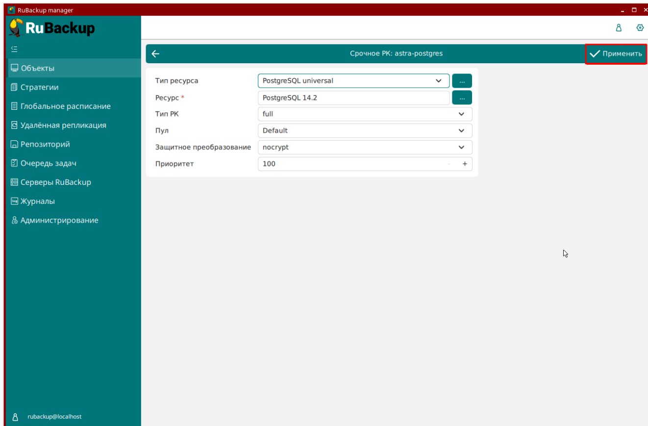
Рисунок 23. Кнопка "Применить"
