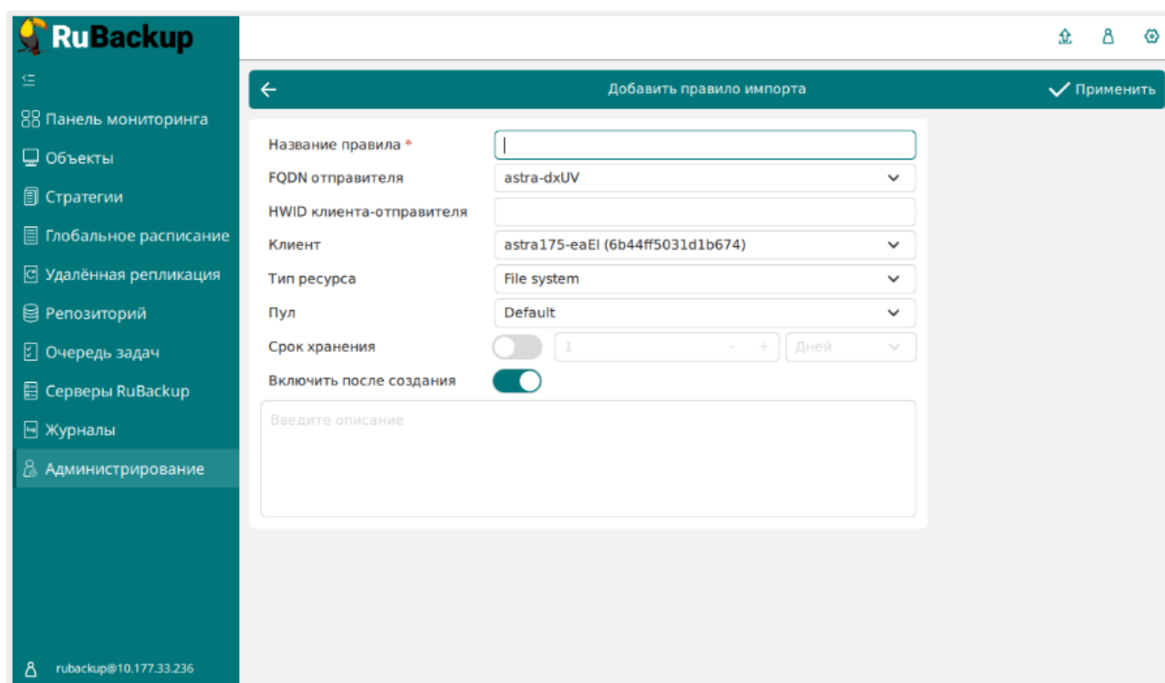
Рисунок 10. Окно добавления правила импорта
