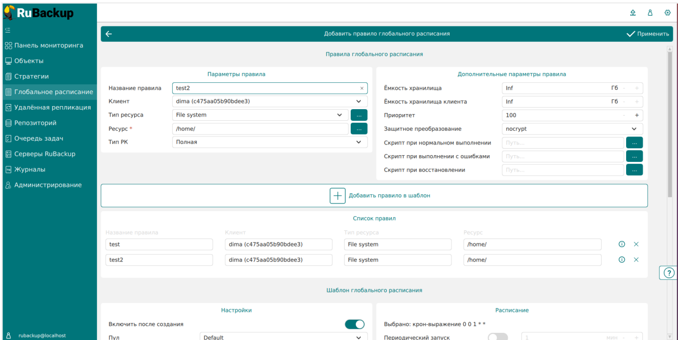
Рисунок 11. Окно «Добавить правило глобального расписания»
