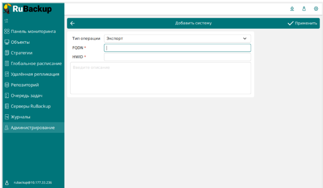
Рисунок 6. Окно добавления СРК-получателя для экспорта РК
