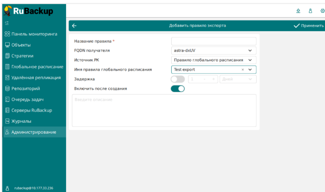
Рисунок 8. Окно добавления правила экспорта
