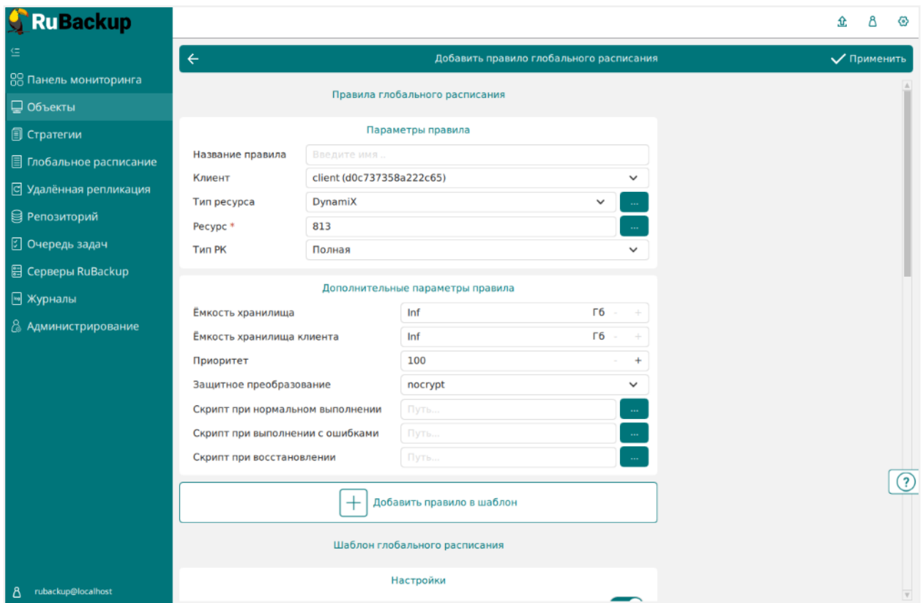
Рисунок 8. Окно создания правила глобального расписания резервного копирования
