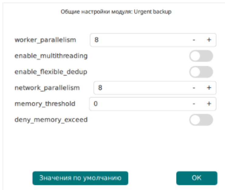
Рисунок 27. Окно Общие настройки модуля (значения по умолчанию)
