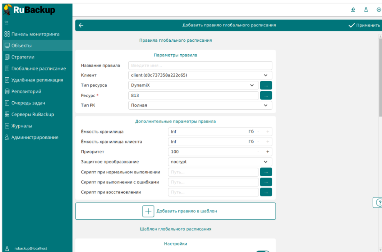
Рисунок 4. Окно создания правила глобального расписания резервного копирования
