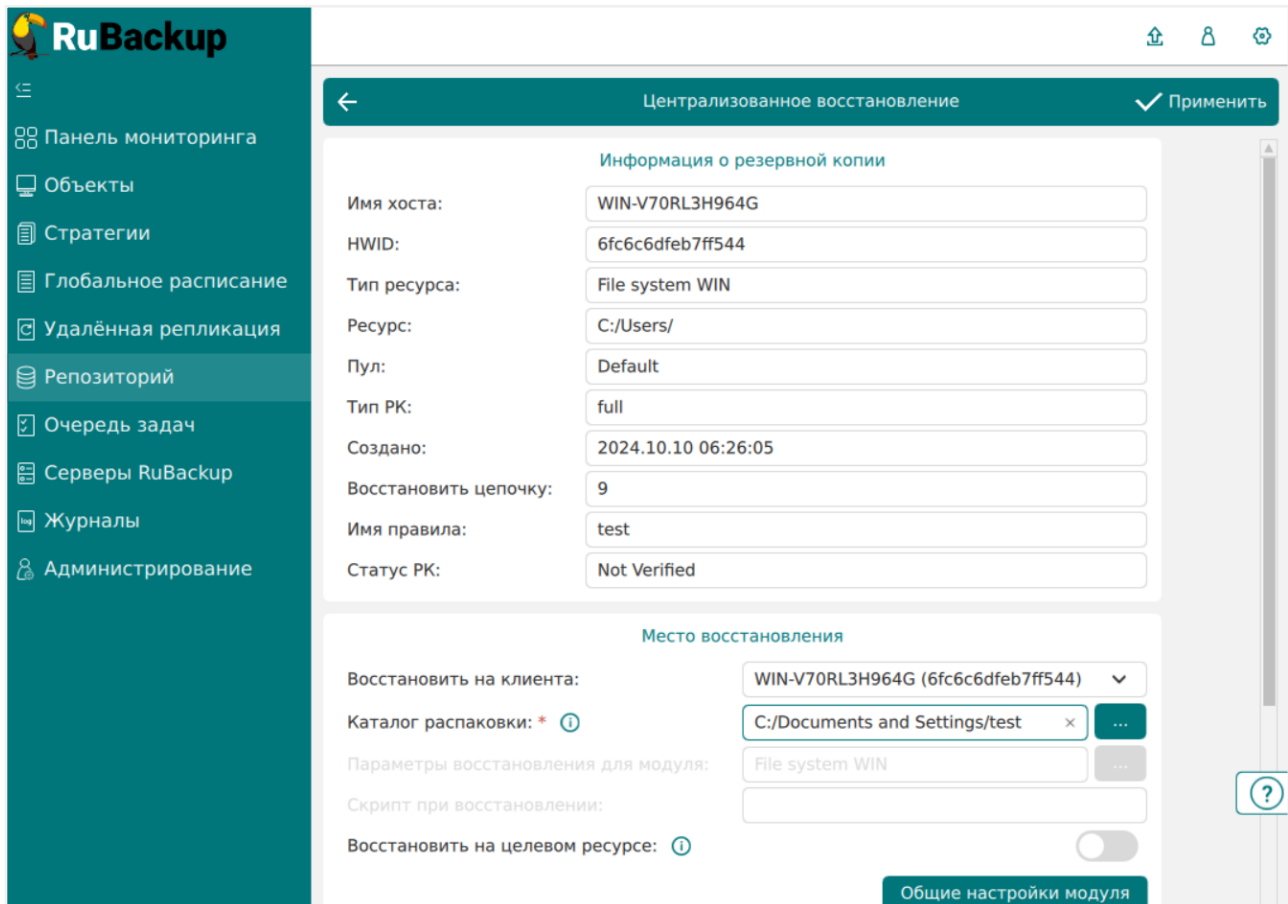
Рисунок 23. Окно Централизованного восстановления VM
