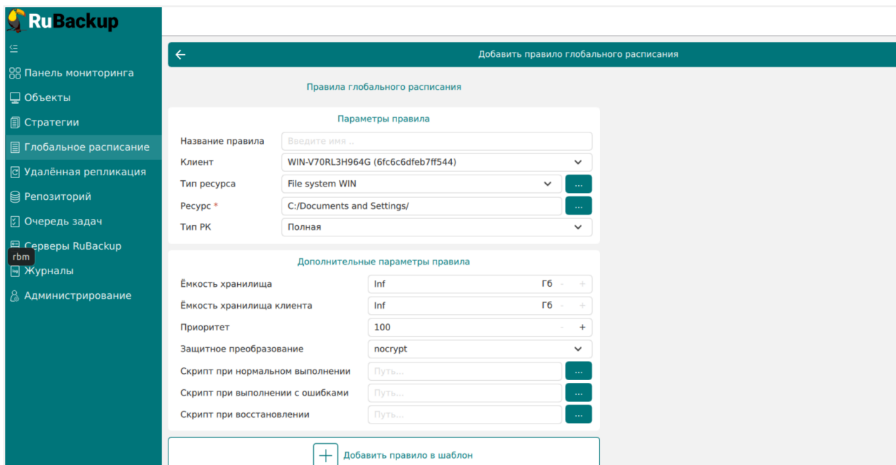
Рисунок 9. Окно создания правила глобального расписания резервного копирования
