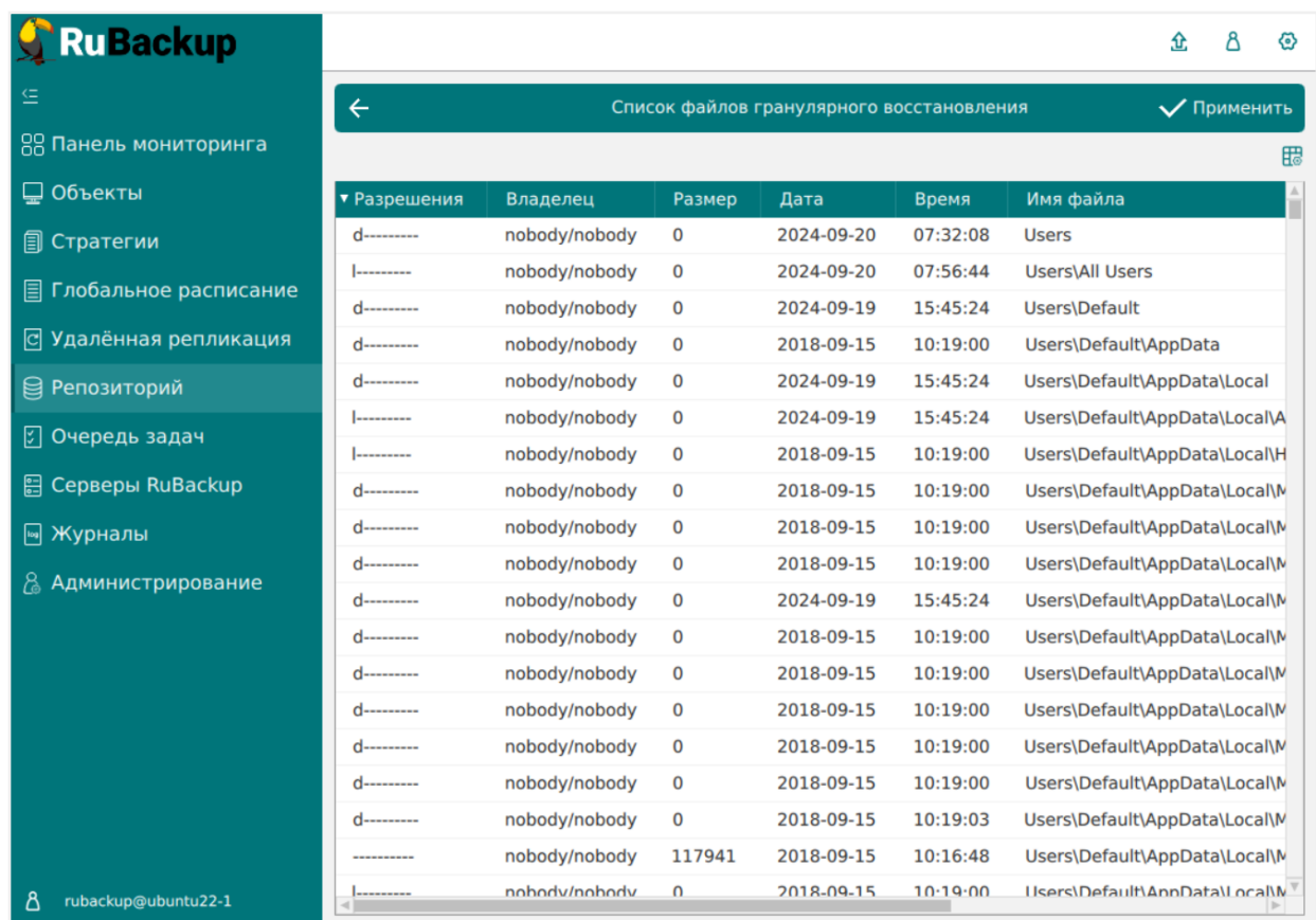
Рисунок 26. Окно выбора ресурсов при гранулярном восстановлении
