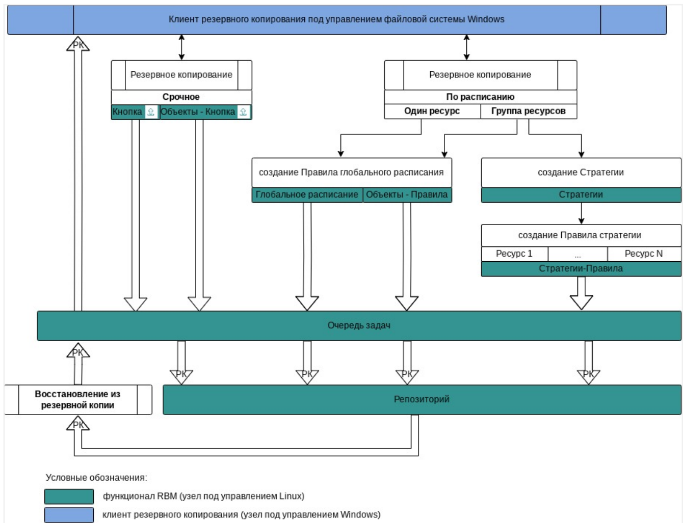
Рисунок 3. Структурная схема резервного копирования и восстановления файловой системы Windows
