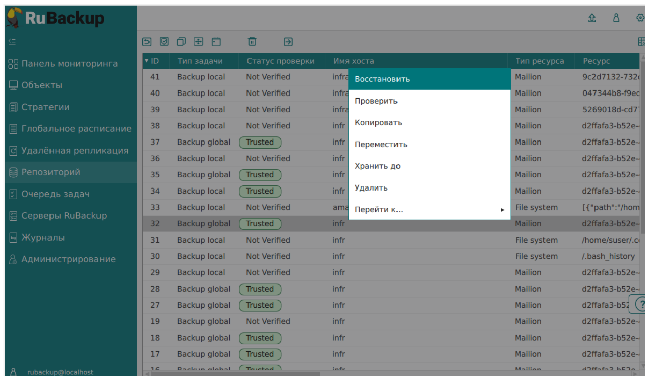
Рисунок 20. Окно раздела «Репозиторий». Восстановление РК
