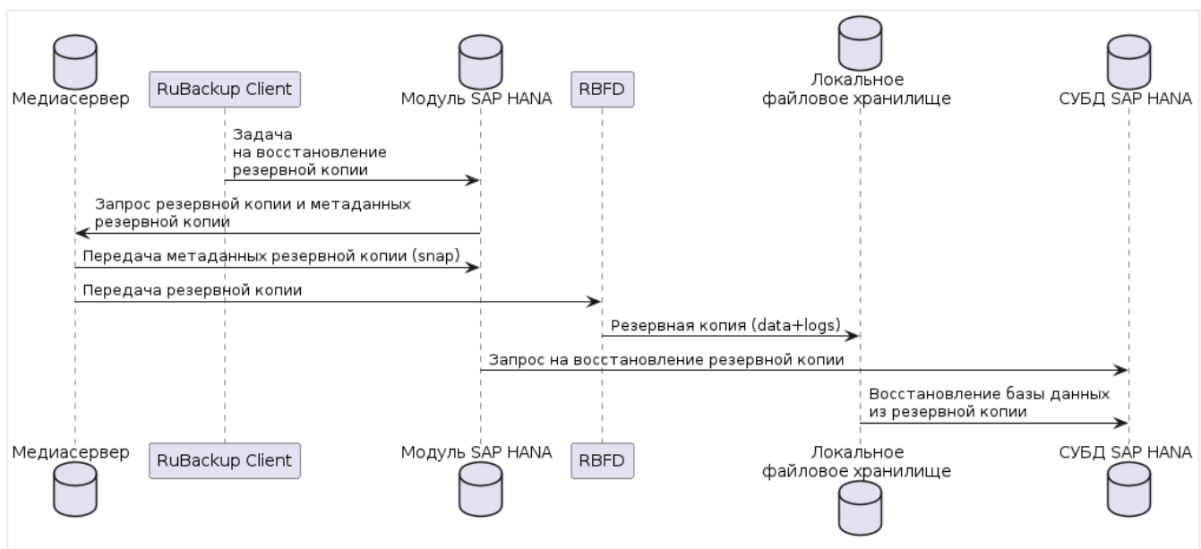
Рисунок 3. Процесс восстановления баз данных СУБД SAP HANA
