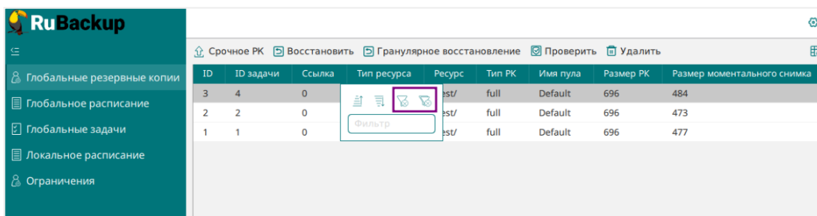
Рисунок 10. Фильтрация данных
