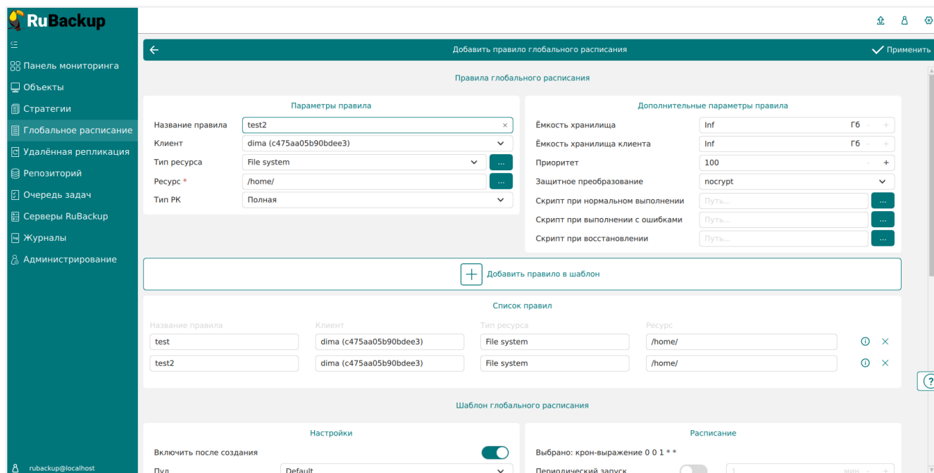
Рисунок 10. Окно «Добавить правило глобального расписания»
