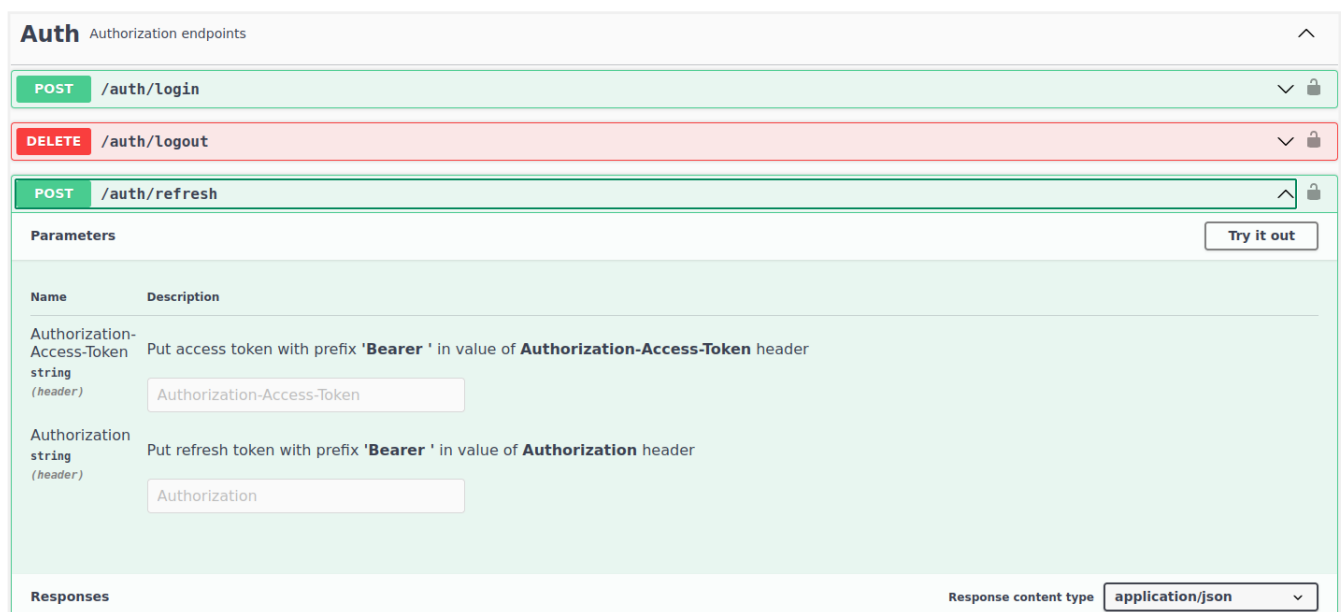
Рисунок 5. Эндпоинт /auth/refresh
